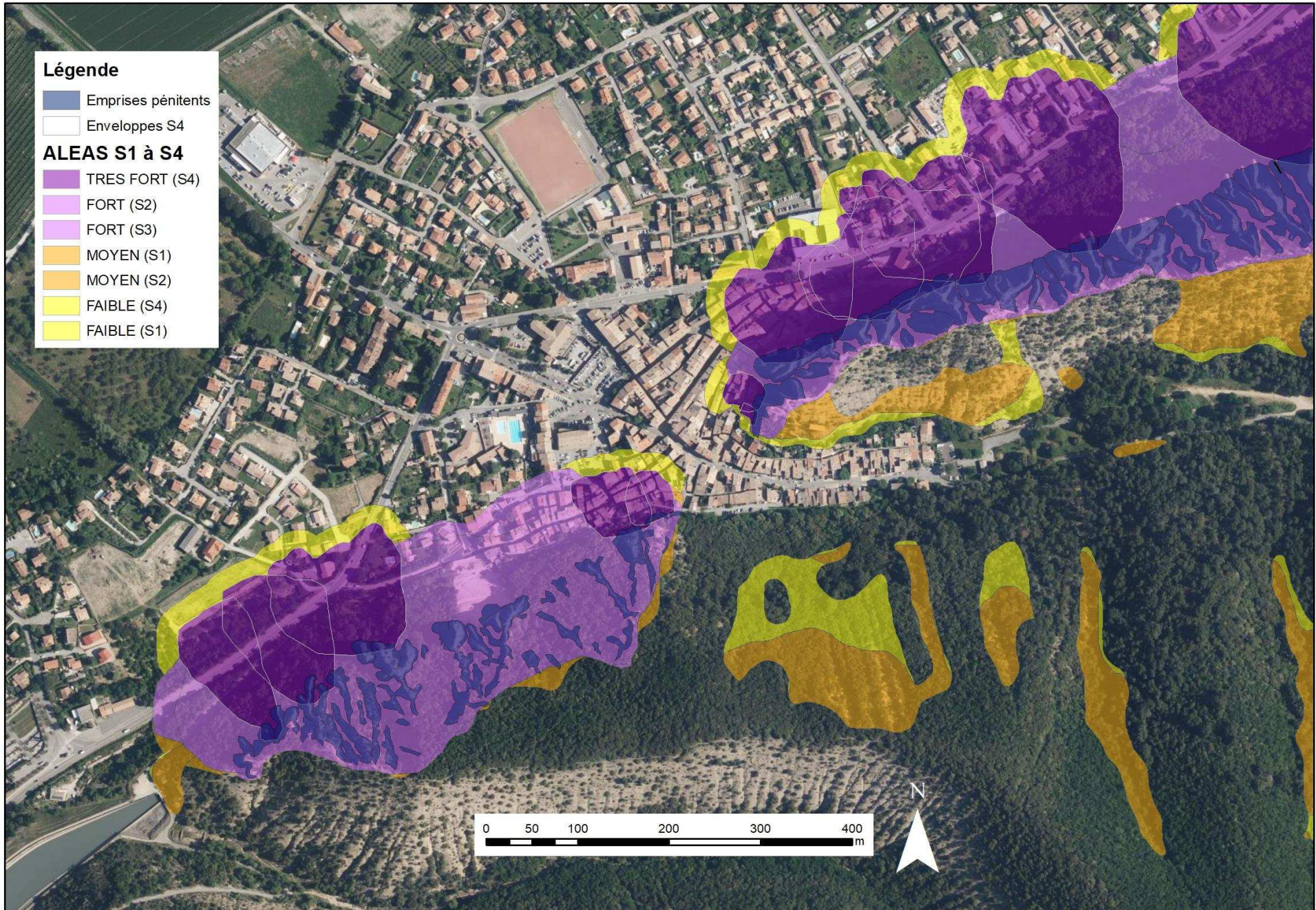
Figure 50 : Cartographie de l'aléa chutes de blocs (planche 1 – fond photo IGN, échelle 1/5000)
