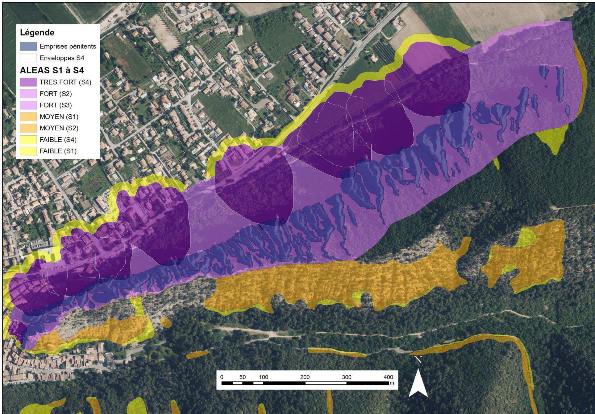
Figure 51 : Cartographie de l'aléa chutes de blocs (planche 2 – fond photo IGN, échelle 1/5000)
